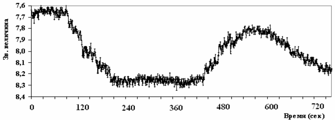
Рис. 4. Фрагмент кривой блеска ГСС Mentor 2 (98029А), наблюдения 07.03.2003г., фильтр V, фазовый угол \varphi = 43^0
